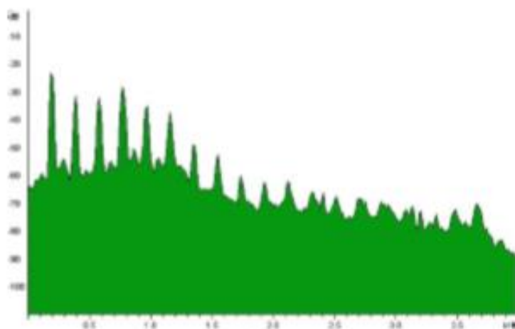
Slika 5. FFT spektral ljudskog glasa (fonacija vokala /A/) (Preuzeto iz Heđever, 2012).
