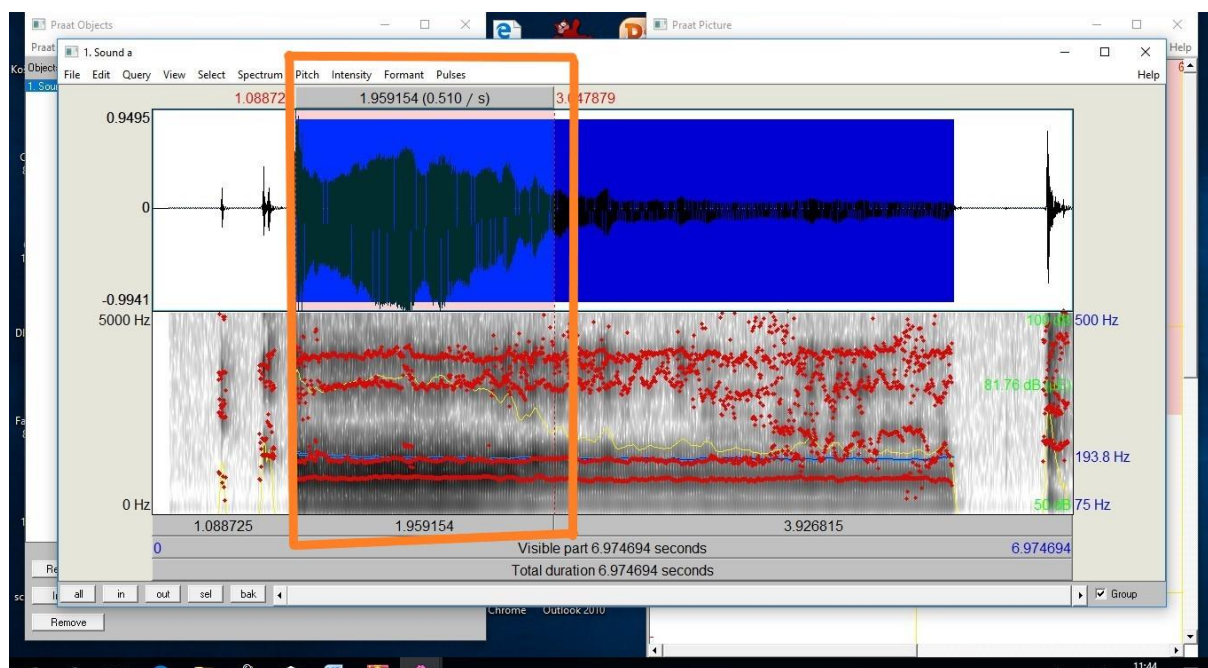
Slika 11. Oscillogram i spektrogram fonacije vokala /A/
