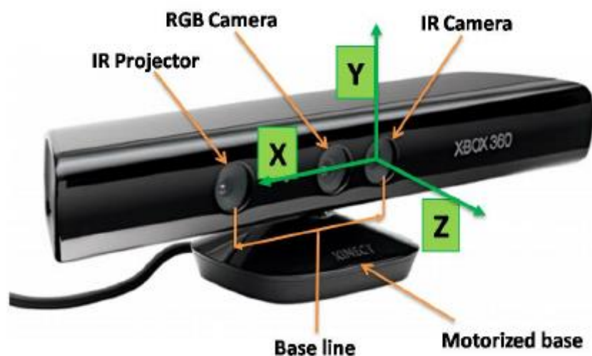
Slika 10 Kinect sistem
